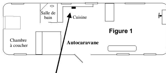
■ Localisation recommandée du détecteur-avertisseur
